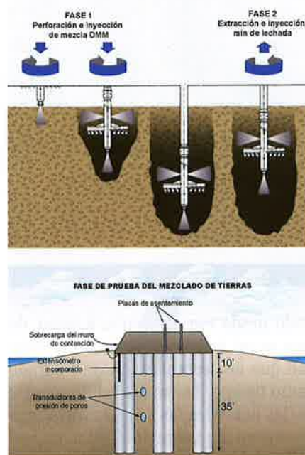
Varias columnas son colocadas en el suelo para proporcionar las propiedades geomecánicas necesarias. En total, se instalaron 1.500 columnas dobles midiendo 13,7 metros.
